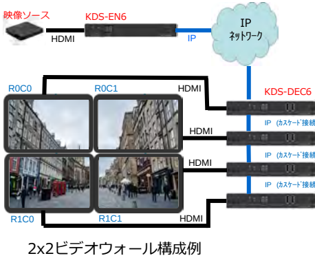
2x2ビデオウォール構成例
