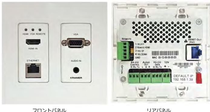
KIT-401T 送信器
