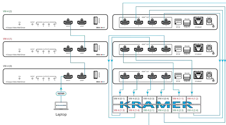
※6x2ビデオウォール構成例
