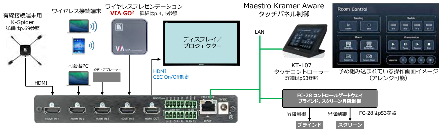
VS-411XS システム構成例
